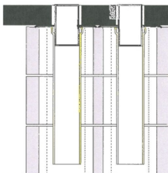
Kopfausbildung Variante 3: Dehnfugenblech und Abdeckplatte Einbau Auflagenblech des Dehnfugenblech unterhalb der Abdeckplatte Einbau Auflagenblech des Dehnfugenblech oberhalb der Abdeckplatte
