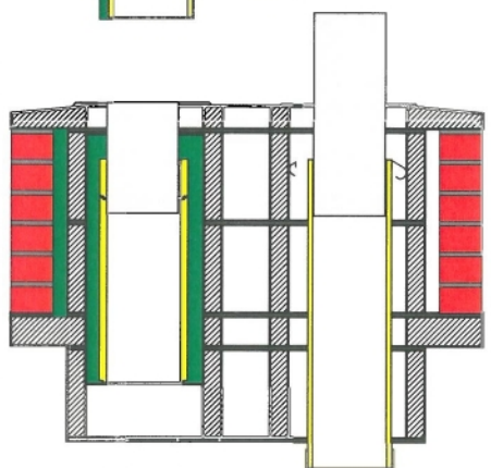
Kopfausbildung Variante 3: Dehnfugenblech und Abdeckplatte Einbau Auflagenblech des Dehnfugenblech unterhalb der Abdeckplatte Einbau Auflagenblech des Dehnfugenblech oberhalb der Abdeckplatte
