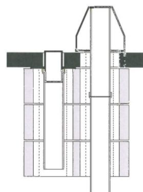
Kopfausbildung Variante 3: Dehnfugenblech und Abdeckplatte Einbau Auflagenblech des Dehnfugenblech unterhalb der Abdeckplatte Einbau Auflagenblech des Dehnfugenblech oberhalb der Abdeckplatte
