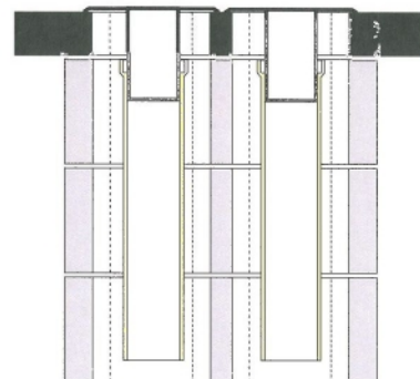
Kopfausbildung Variante 3: Dehnfugenblech und Abdeckplatte Einbau Auflagenblech des Dehnfugenblech unterhalb der Abdeckplatte Einbau Auflagenblech des Dehnfugenblech oberhalb der Abdeckplatte
