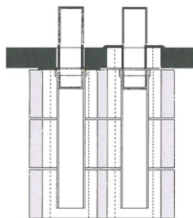
Kopfausbildung Variante 3: Dehnfugenblech und Abdeckplatte Einbau Auflagenblech des Dehnfugenblech unterhalb der Abdeckplatte Einbau Auflagenblech des Dehnfugenblech oberhalb der Abdeckplatte
