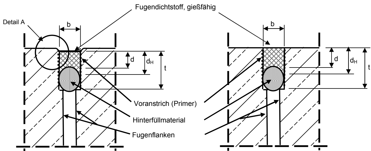
Befahrbare Fugenkonstruktion
