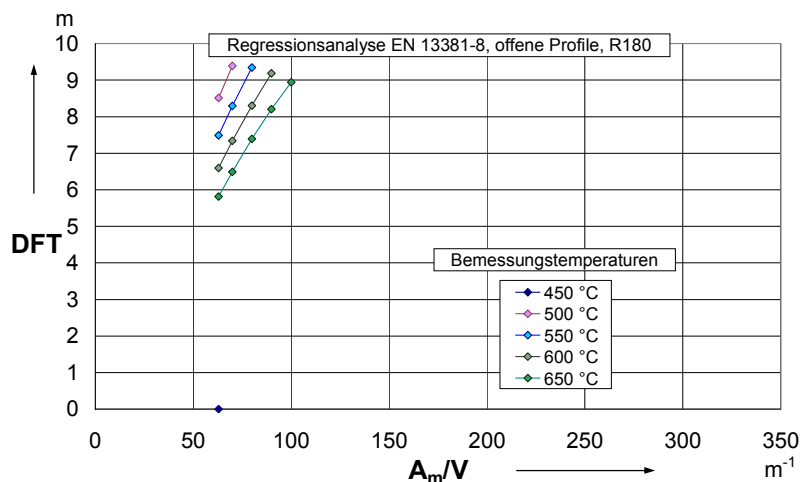
Anlage 1, Tabelle 7: Stützen, offene Profile (H und I Profile)
