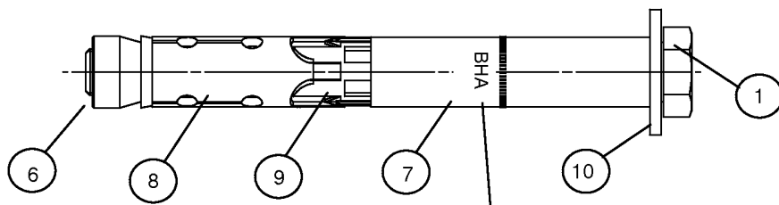
Schraubenversion Typ S BHA 10 - 32
