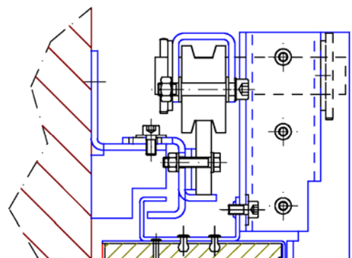
Stahlhangrolle auf Flachstahllaufschiene als Doppelaufwerk (Schiebergewicht bis 800 kg)
