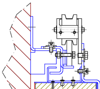
Stahlhangrolle auf Flachstahllaufschiene (Schiebergewicht bis 400 kg)
