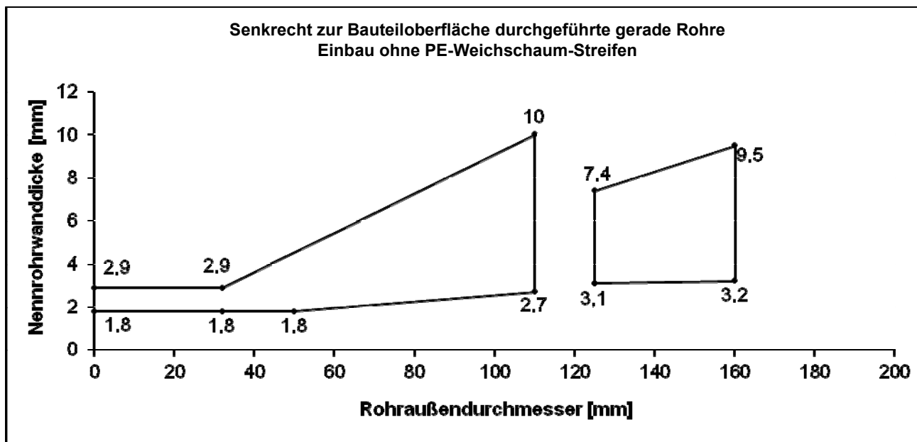
Bild 9 – EI 90-U/U (Deckeneinbau)
