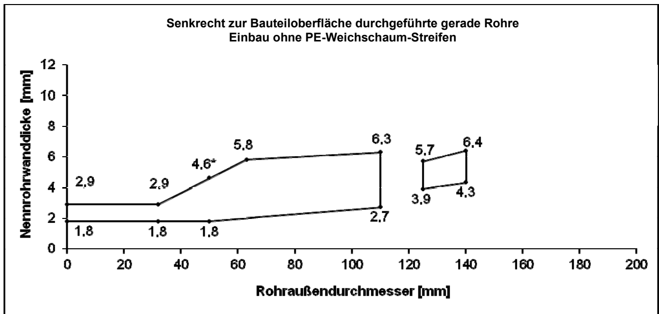
Bild 6 – EI 90-U/U (Wandebau)
