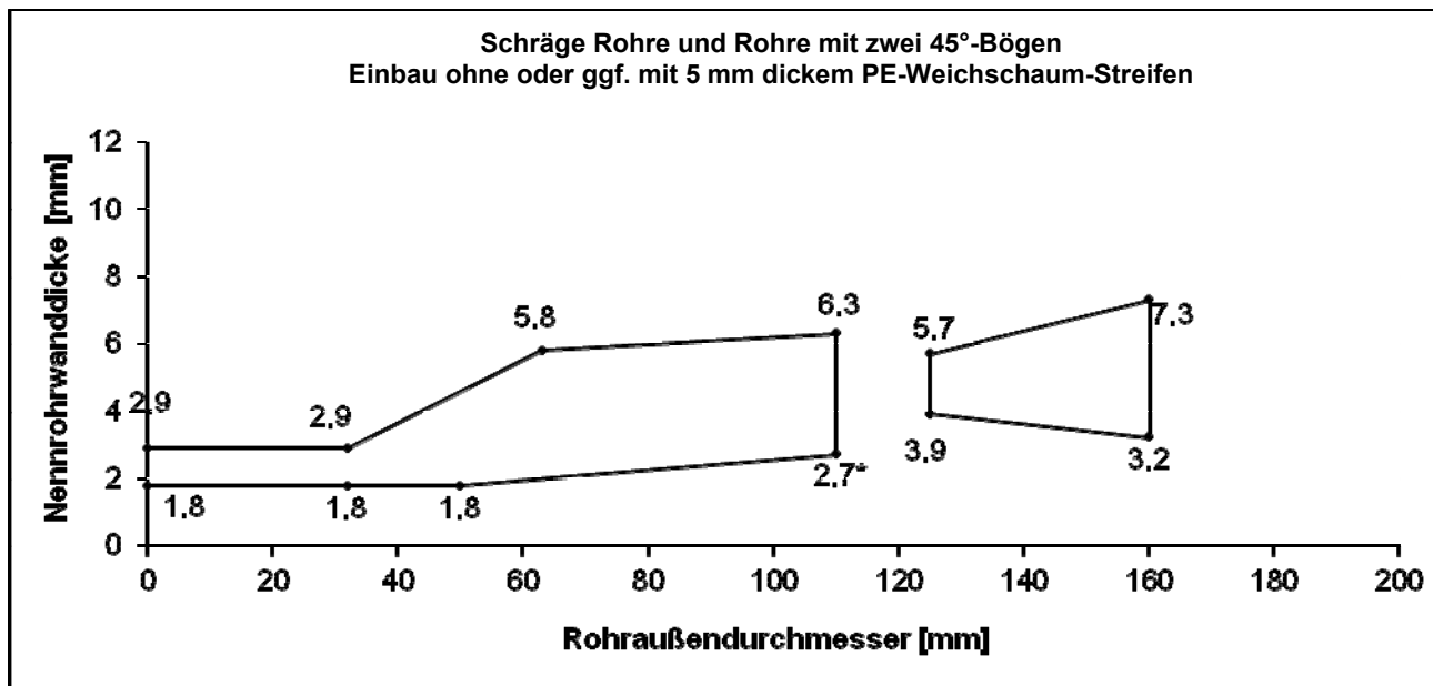
Bild 8 – EI 90-U/C (Wandebau)
