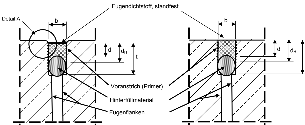
Befahrbare Fugenkonstruktion
