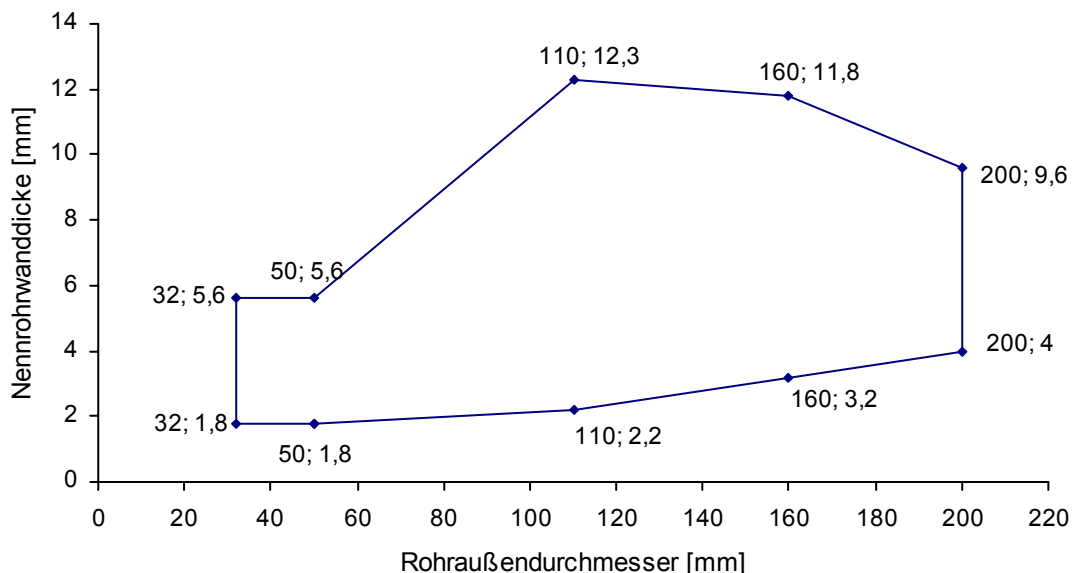
Bild 6: Rohre gemäß Rohrgruppe A (PVC): Einbau in Massivdecken; d_b \geq 150 mm; Feuerwiderstandsklasse EI 120-U/C
