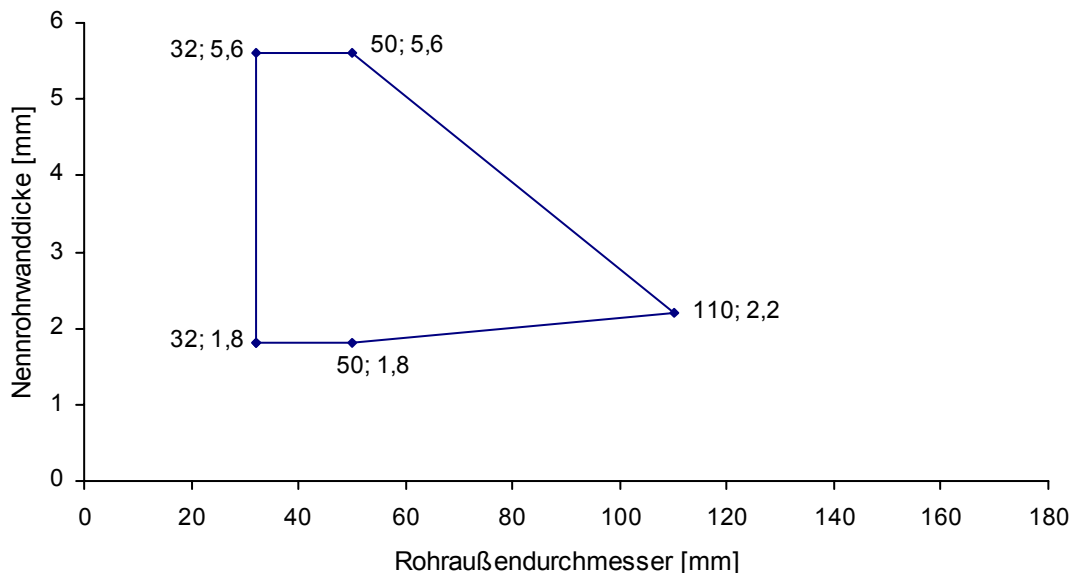
Bild 2: Rohre gemäß Rohrgruppe A (PVC): Einbau in leichte Trennwände; d_w \geq 100 mm; Feuerwiderstandsklasse EI 120–U/C
