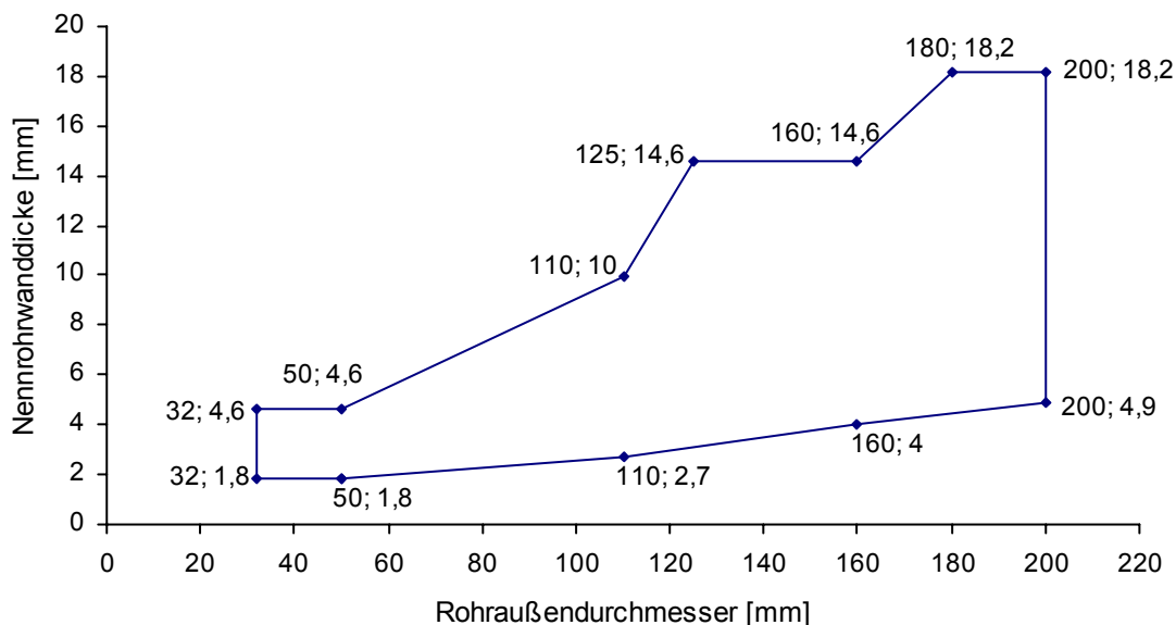
Bild 12: Rohre gemäß Rohrgruppe B (PE-HD): Einbau in Massivdecken; d_D \geq 300 mm; Feuerwiderstandsklasse EI 120-U/C
