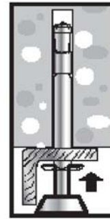
oder Einschlagen mit einem Setzwerkzeug
