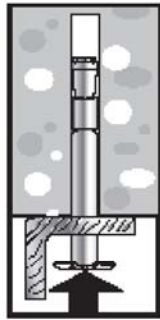
Setzen des Dübels durch das Anbauteil
