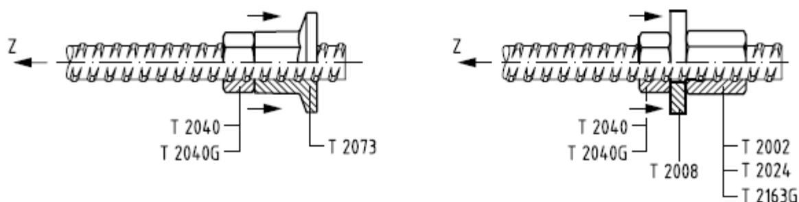
Bild 9: GEWI®-Verankerung bei Druckbeanspruchung
