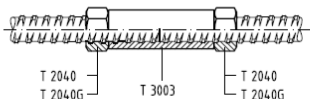
Bild 2: GEWI®-Muffenstoß-lang (SW)
