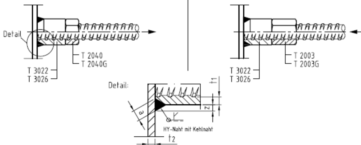
Bild 7: GEWI®-Schweißanschluß
