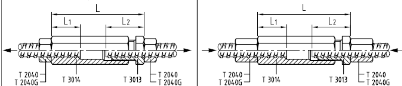
Bild 6: GEWI®-Spannmuffenstoß
