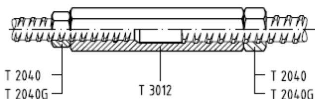
Bild 4: GEWI®-Reduziermuffenstoß-lang (SW)
