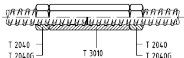
Bild 3: GEWI®-Reduziermuffenstoß
