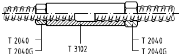
Bild 4: GEWI®-Reduziermuffenstoß-lang (SW)
