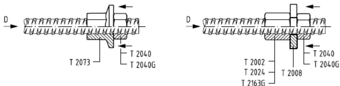
Bild 10: GEWI®-Verankerung bei Wechselbeanspruchung
