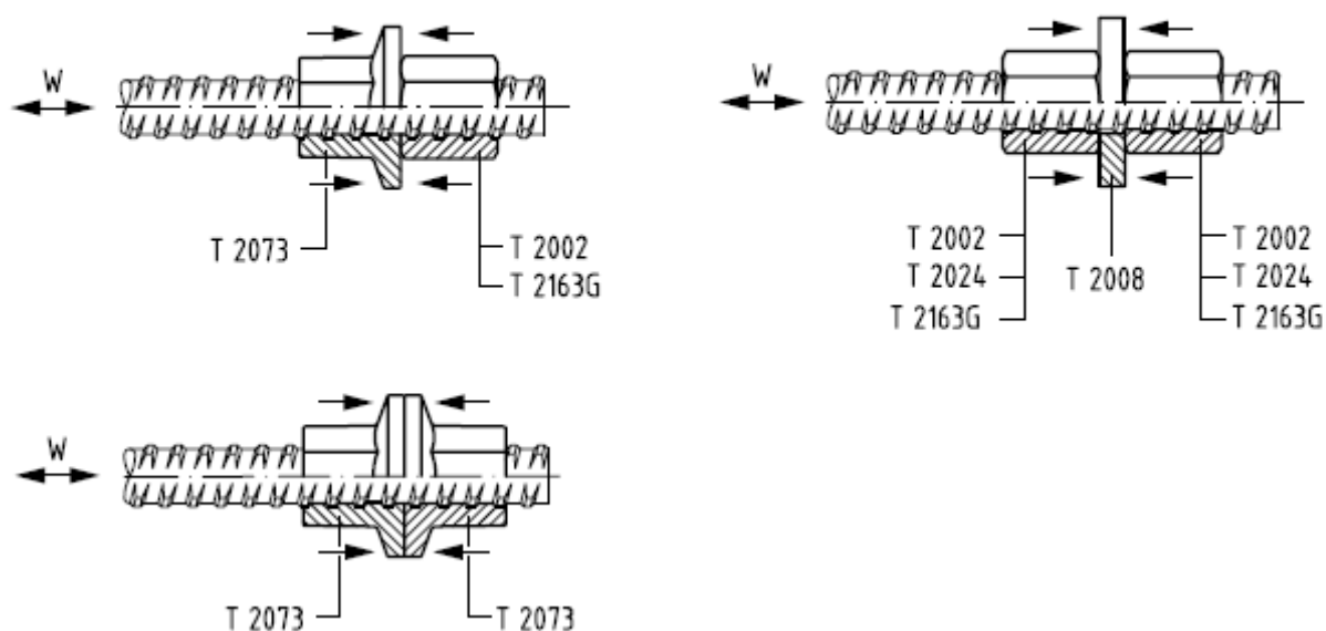
Bild 10: GEWI®-Verankerung bei Wechselbeanspruchung
