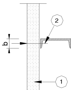
BILD 1 Stahl-Auflager
