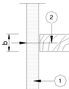
BILD 2 Holz-Auflager
