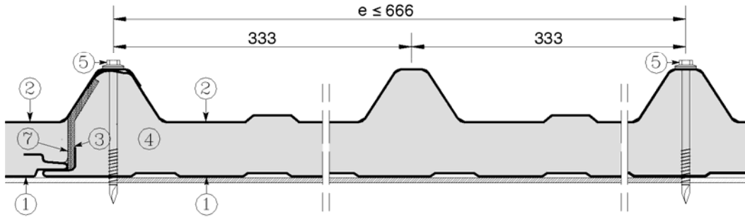
Obergurtbefestigung
