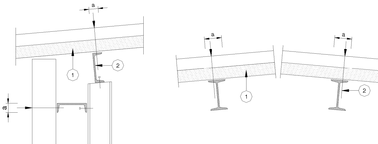
BILD 4 Traufpunkt
