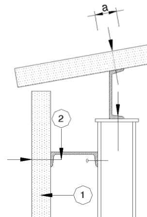
BILD 6 Traufpunkt Wandpaneel
