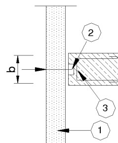
BILD 3 Beton-Auflager
