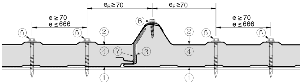
Untergurtbefestigung
