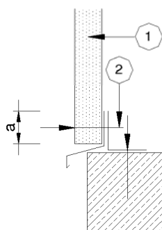
BILD 4 Fußpunkt Wandpaneel aufgesetzt
