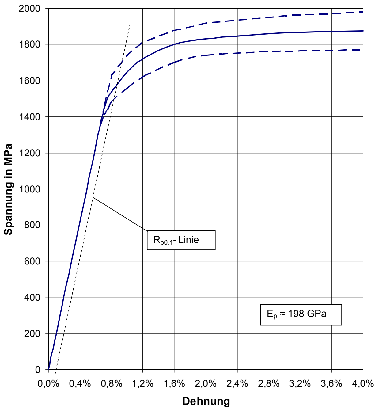
Bild 2: Spannungs-Dehnungs-Linie
