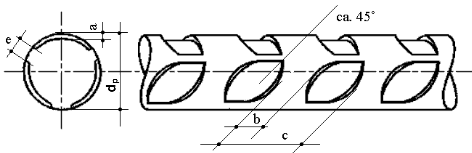
Bild 1: sonderprofilierter Spannstahl
