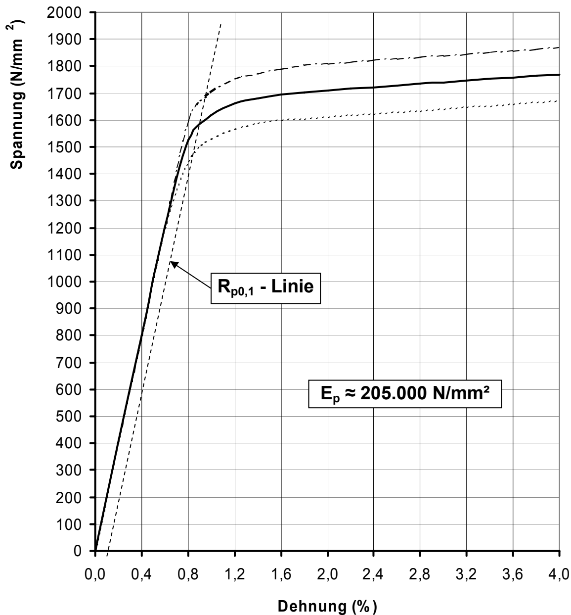
Bild 2: Spannungs-Dehnungs-Linie
