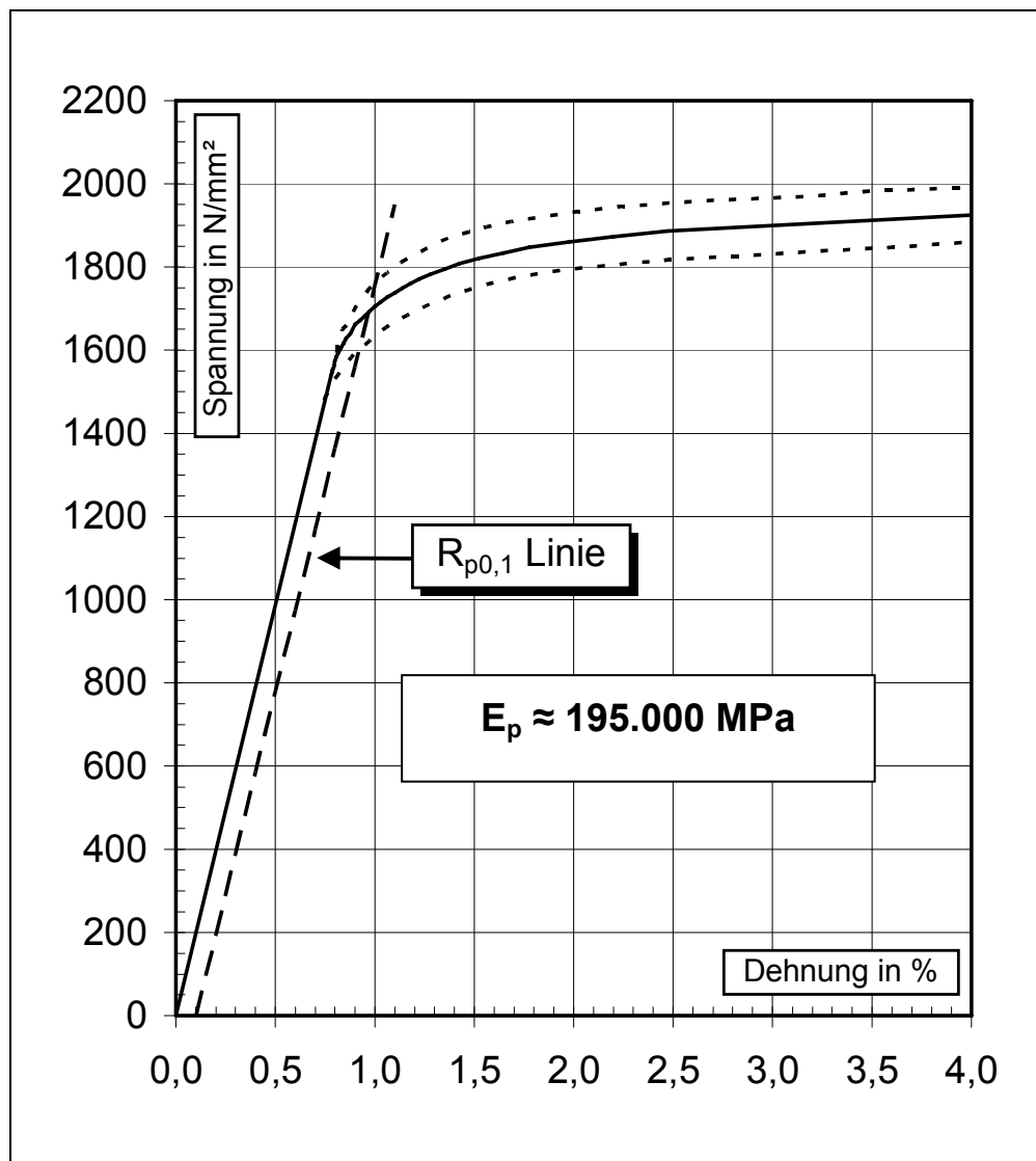
Bild 2: Spannungs - Dehnungslinie
