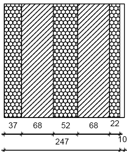
Schnitt B - B
