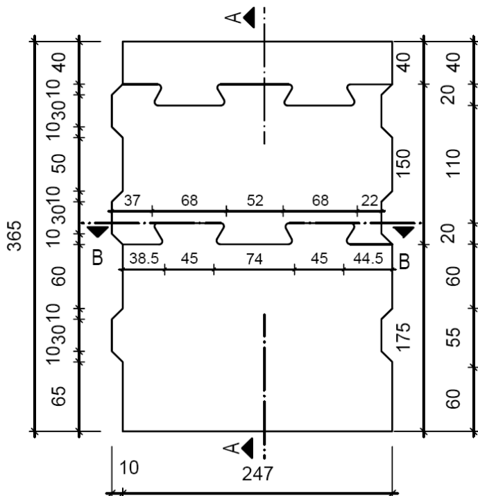
Draufsicht
