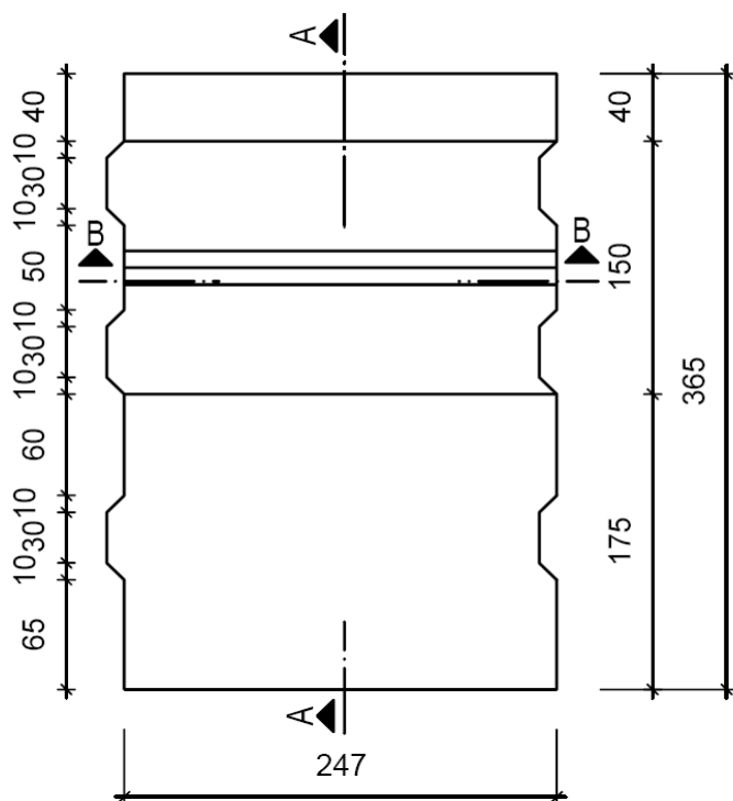
Draufsicht
