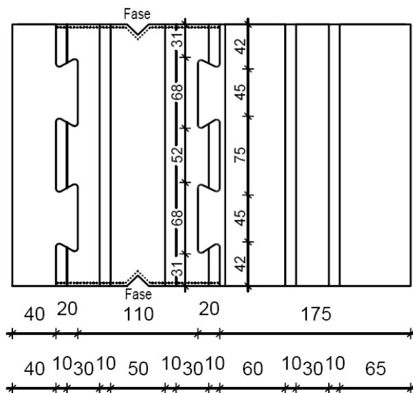
Ansicht u. Produktionslage
