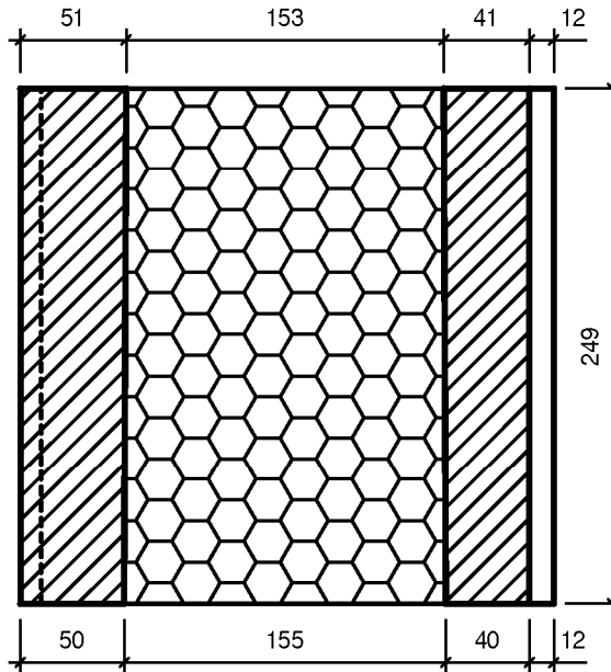
Schnitt A-A
