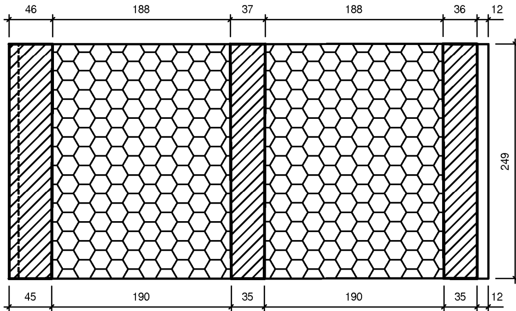
Schnitt A-A
