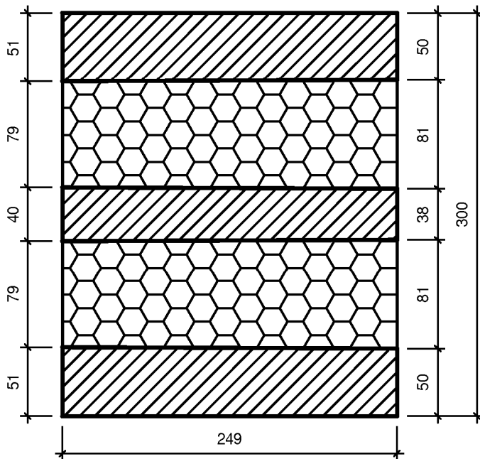
Schnitt B-B
