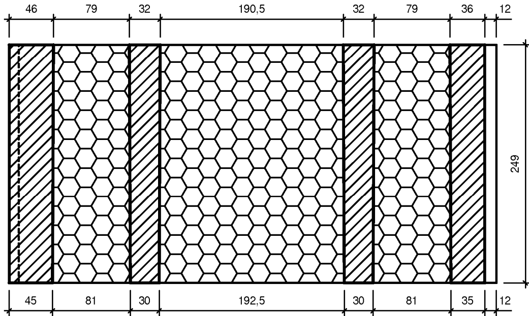
Schnitt A-A
