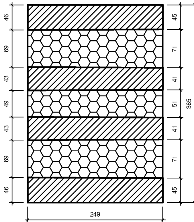
Schnitt B-B
