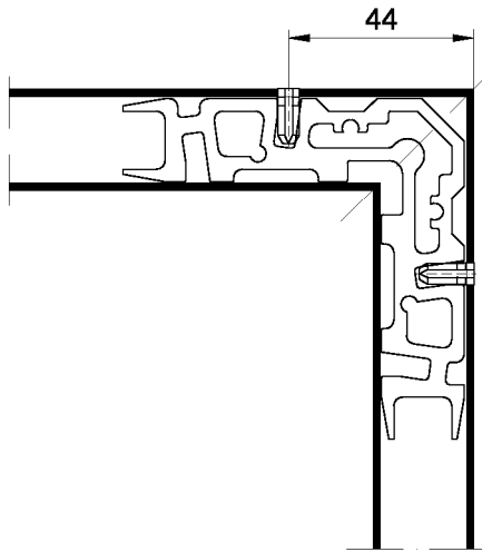
Einzelheit "X"
