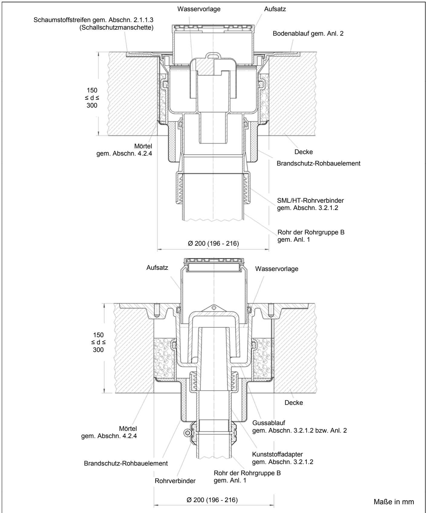
Rohrabschottung "DALLMER Ablauf mit Brandschutzelement Nr. ..." der Feuerwiderstandsklassen R 120, R 90, R 60 oder R 30 nach DIN 4102-11
