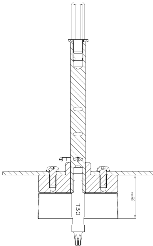
Bild 4.3: ejotherm STR U 2G Montagetool Typ "L" für Dämmstoffdicken ab 100 mm
