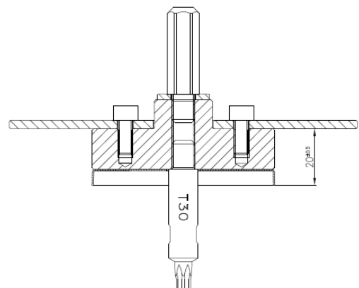
Bild 4.2: ejotherm STR U Montagetool Typ "S" für Dämmstoffdicken ab 80 mm
