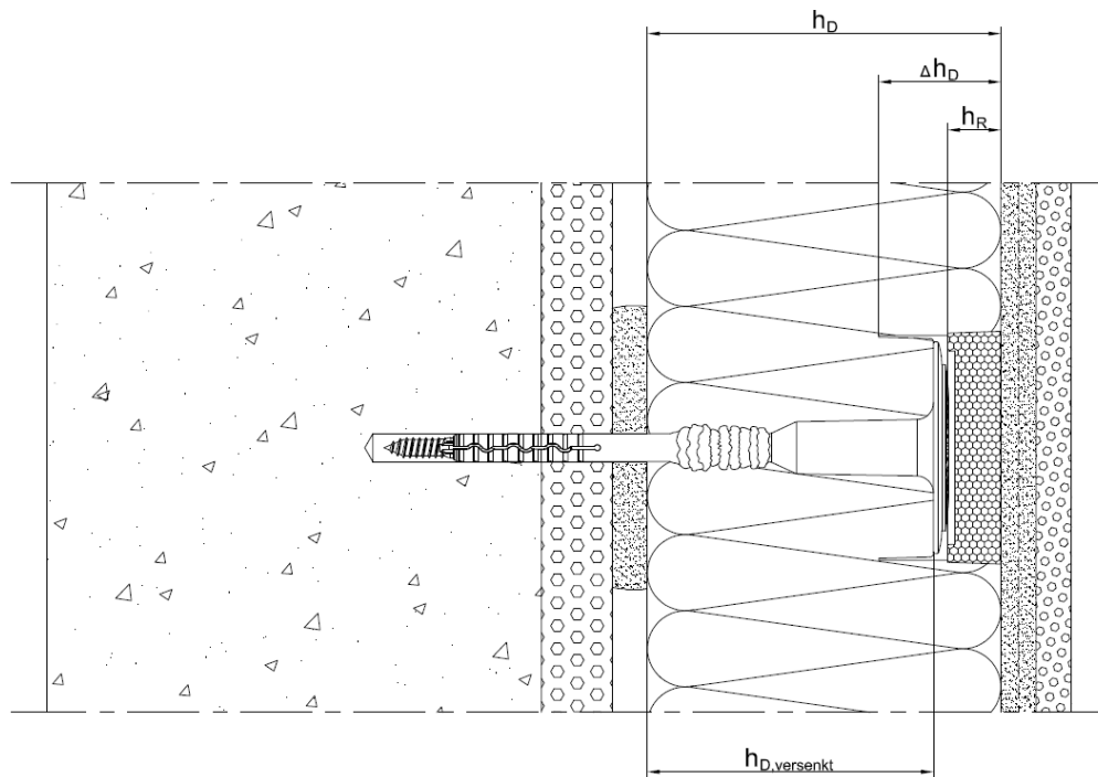
Bild 5.1: ejotherm STR U und ejotherm STR U 2G (versenkte Montage)
