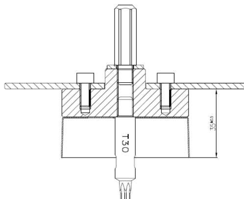
Bild 4.1: ejotherm STR U Montagetool Typ "L" für Dämmstoffdicken ab 100 mm
