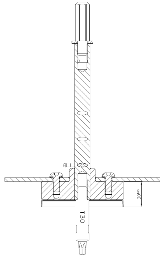
Bild 4.4: ejotherm STR U 2G Montagetool Typ "S" für Dämmstoffdicken ab 80 mm
