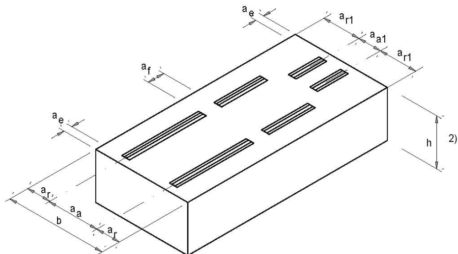
Mindestabstände und Mindestbauteilabmessungen ohne konstruktive Bewehrung Tabelle 11:
