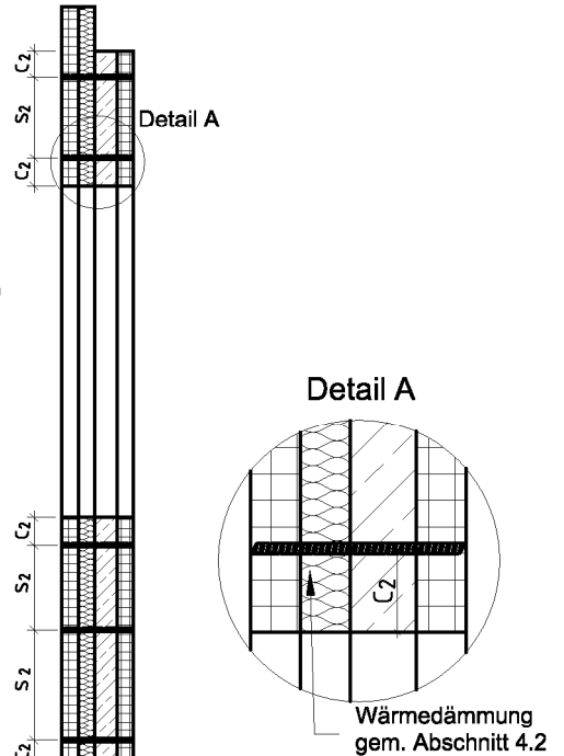
Schnitt B-B Elementwand:
