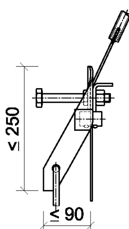
Seitenansicht
