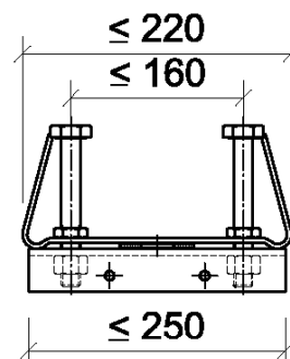
Draufsicht
