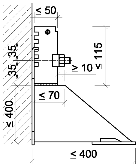
Seitenansicht
