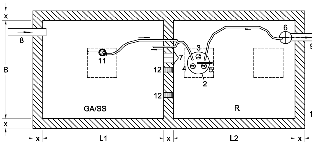
Draufsicht
