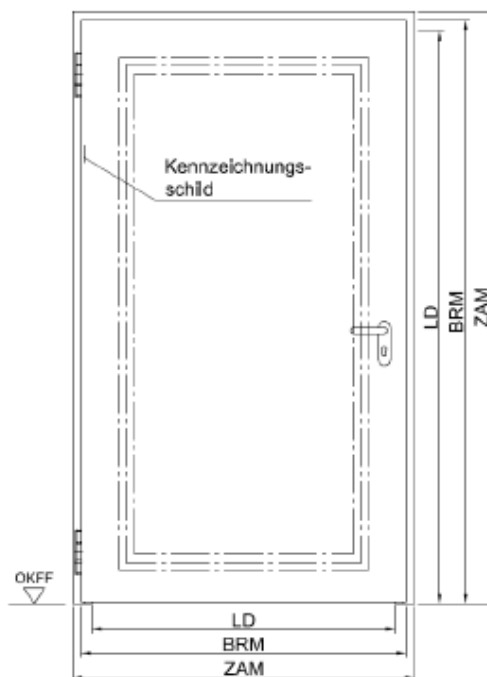
Dargestellt: Gangflügel DIN links, Gangflügel DIN rechts spiegelbildlich
