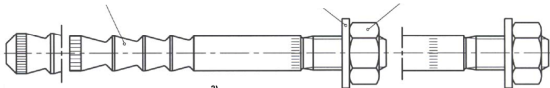
Anchor rod VMZ-IG 2)
