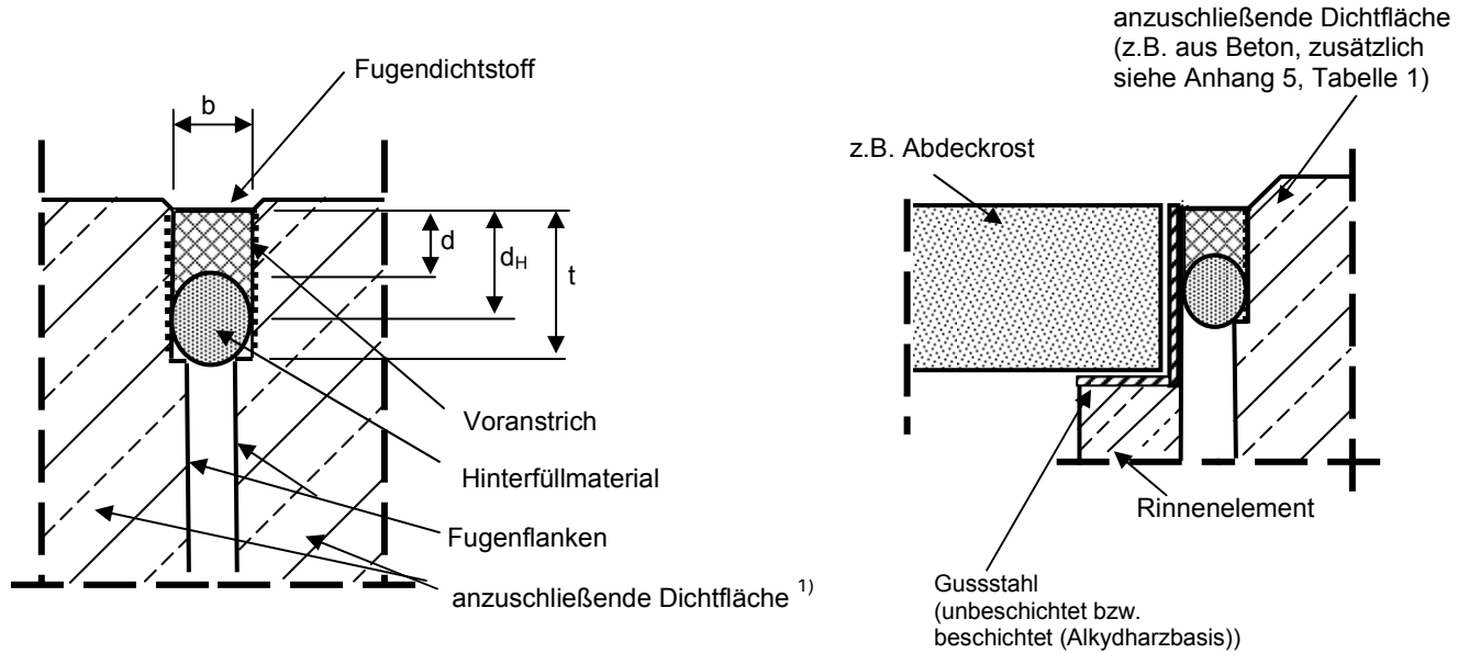
Bild 1: befahrbare Fugenausbildung
