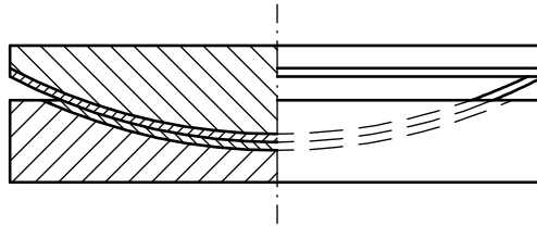
Unverschieblich durch Gleitfläche (3.2). Abb. A.2 - mageba ROBO ® SLIDE L2 Kalottenlager
