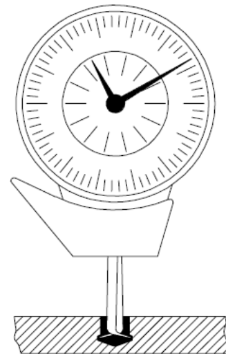
2. Schnelltaster (Messuhr)
