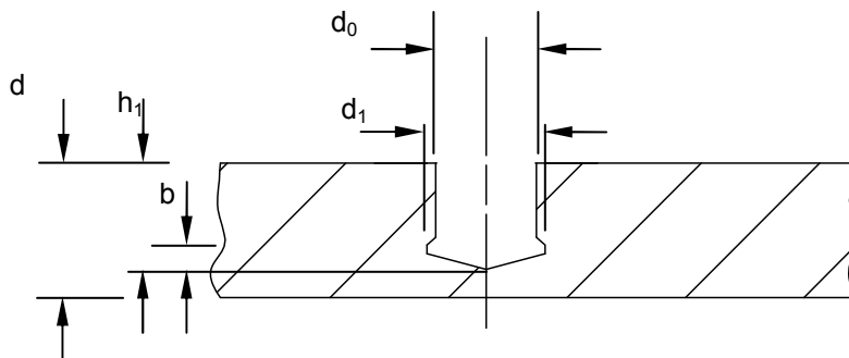
2. Bohrlochgeometrie
