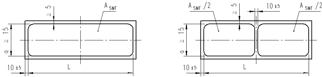
Abb. B.4 - Beispiele für gekammerte SMF-Platten für Führungen
