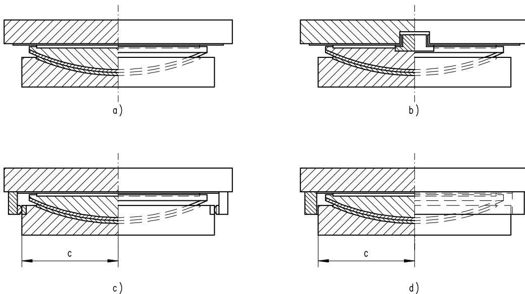
Unverschieblich durch Gleitfläche (3.2). Abb. A.2 - FIP SMF Kalottenlager
