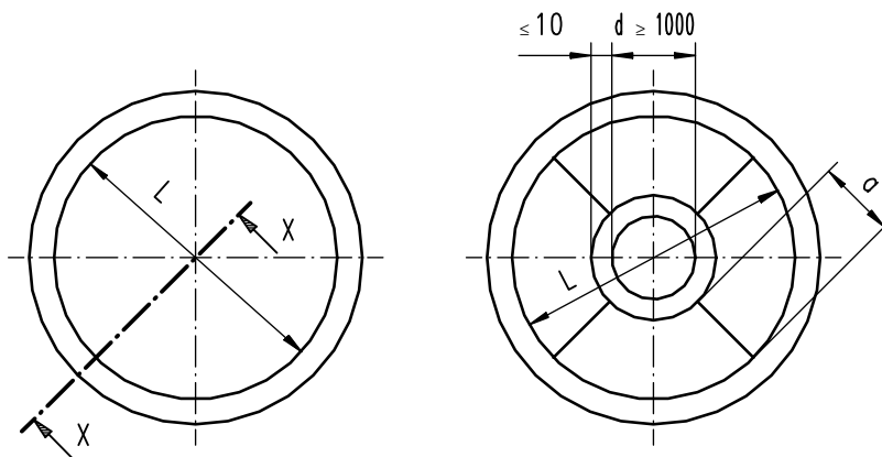
Abb. B.3 - Unterteilung gekammerter SMF-Platten für kugelige Gleitflächen
