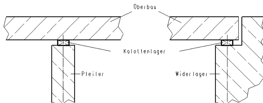
Abb. A.1 - Zusammenbau eines geführten und allseits beweglichen FIP SMF Kalottenlagers und vorgesehener Verwendungszweck (Beispiel)
