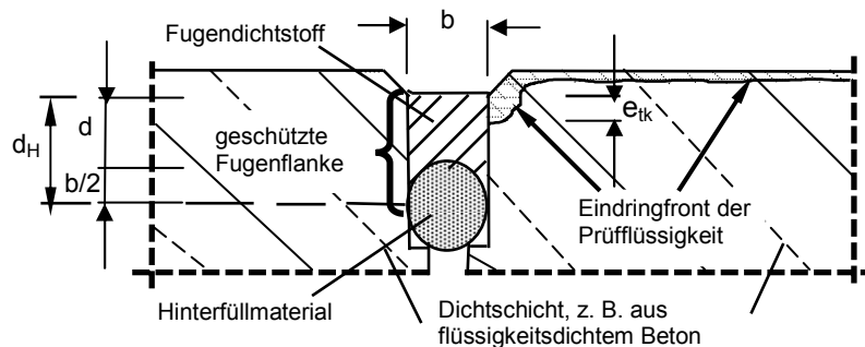
Bild 1: Umläufigkeitsverhalten im Bereich des eingebauten Fugenabdichtungssystems 1)
