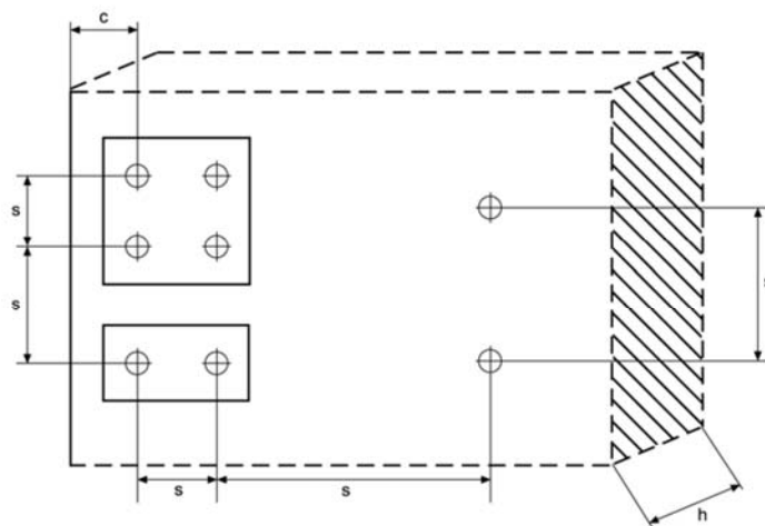
Anordnung Randabstände und Achsabstände in Beton
