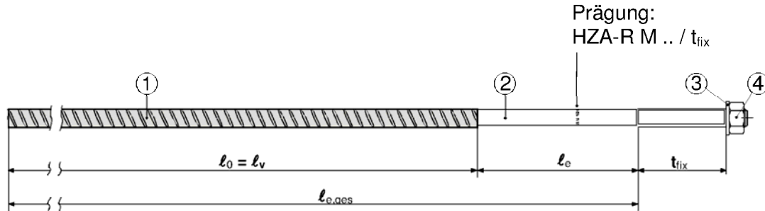
Bild 11: Zuganker HZA-R
