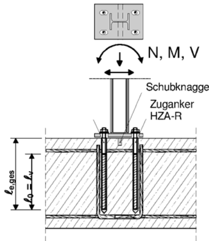
Bild 6: Übergreifungsstoß einer biegebeanspruchten Stütze an ein Fundament
