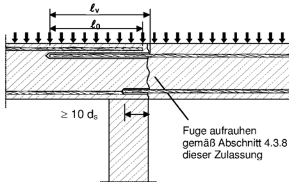
Bild 1: Übergreifungsstoß für Bewehrungsanschlüsse von Platten und Balken
