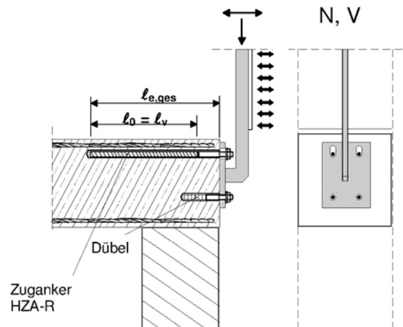
Bild 7: Übergreifungsstoß für die Verankerung von Geländerpfosten
