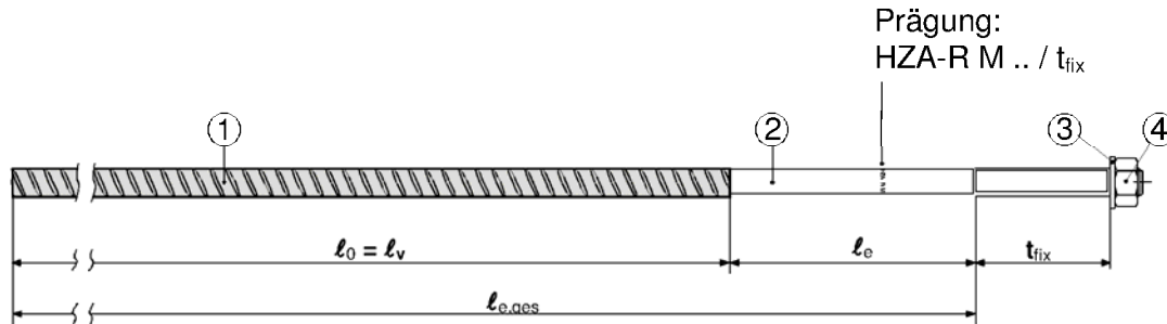
Bild 11: Zuganker HZA-R
