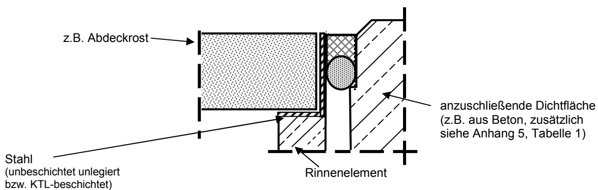
Bild 2: Stahl (unbeschichtet unlegiert bzw. KTL-beschichtet 1) )
