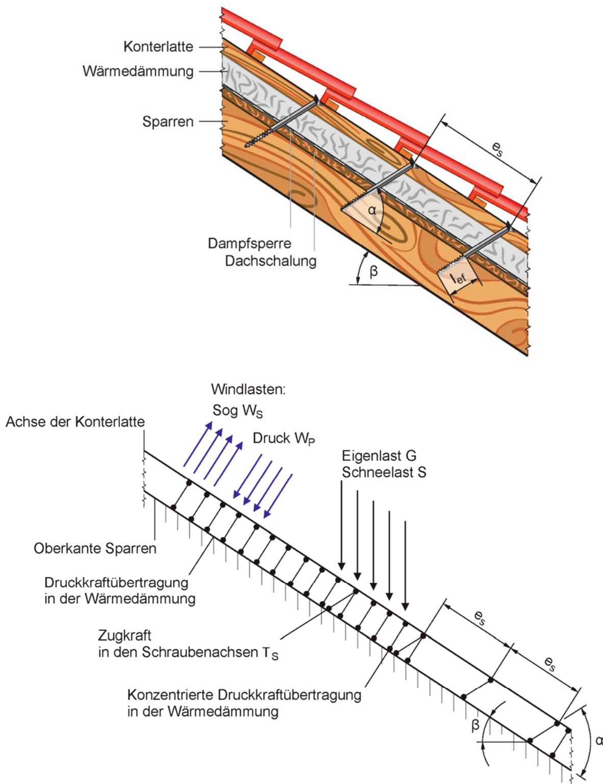
Abbildung 2.1: Befestigung von Aufdach-Dämmsystemen auf Sparren- Statisches Modell für parallel angeordnete Schrauben
