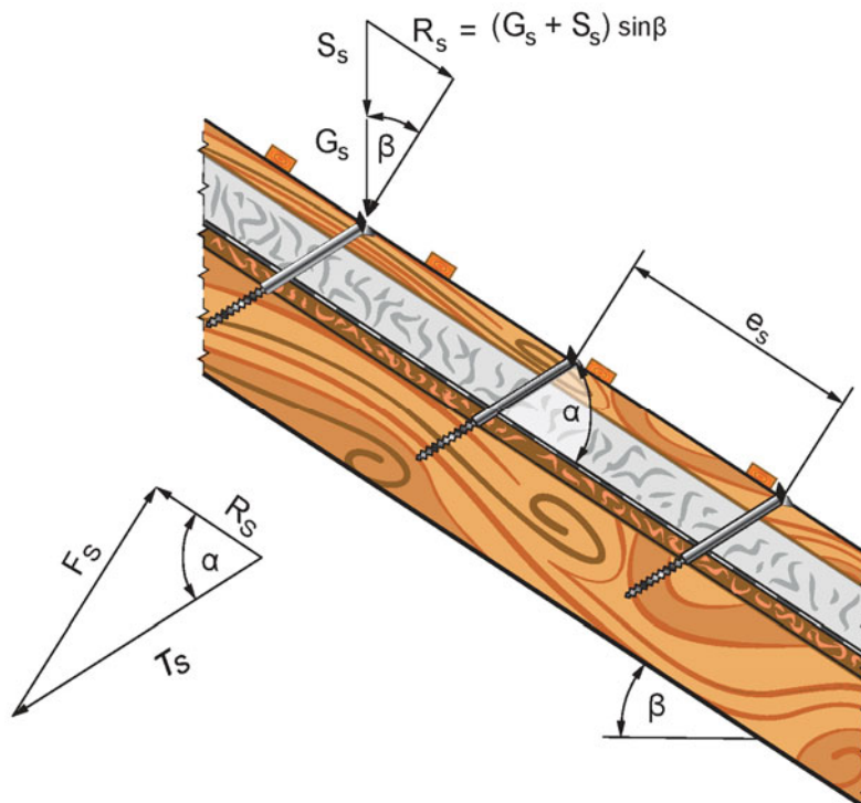
Abbildung 2.3: Einzellasten F_s rechtwinklig zu den Konterlatten, Lastangriff im Bereich des Schraubenkopfes
