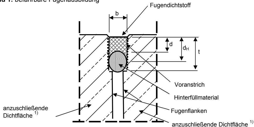
Bild 1: befahrbare Fugenausbildung
