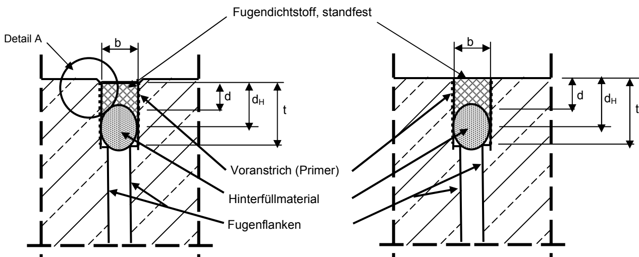
Befahrbare Fugenkonstruktion
