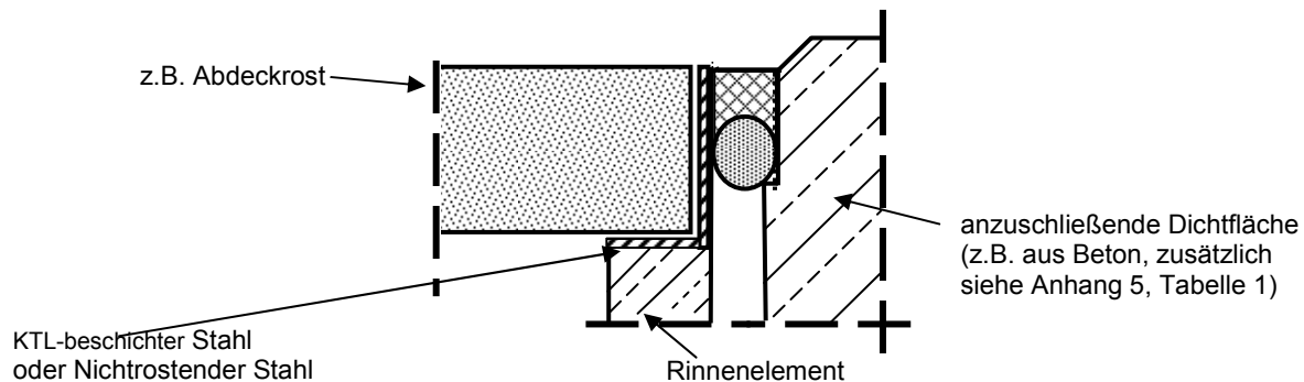
Bild 2: KTL-beschichteter Stahl 1) oder Nichtrostender Stahl
