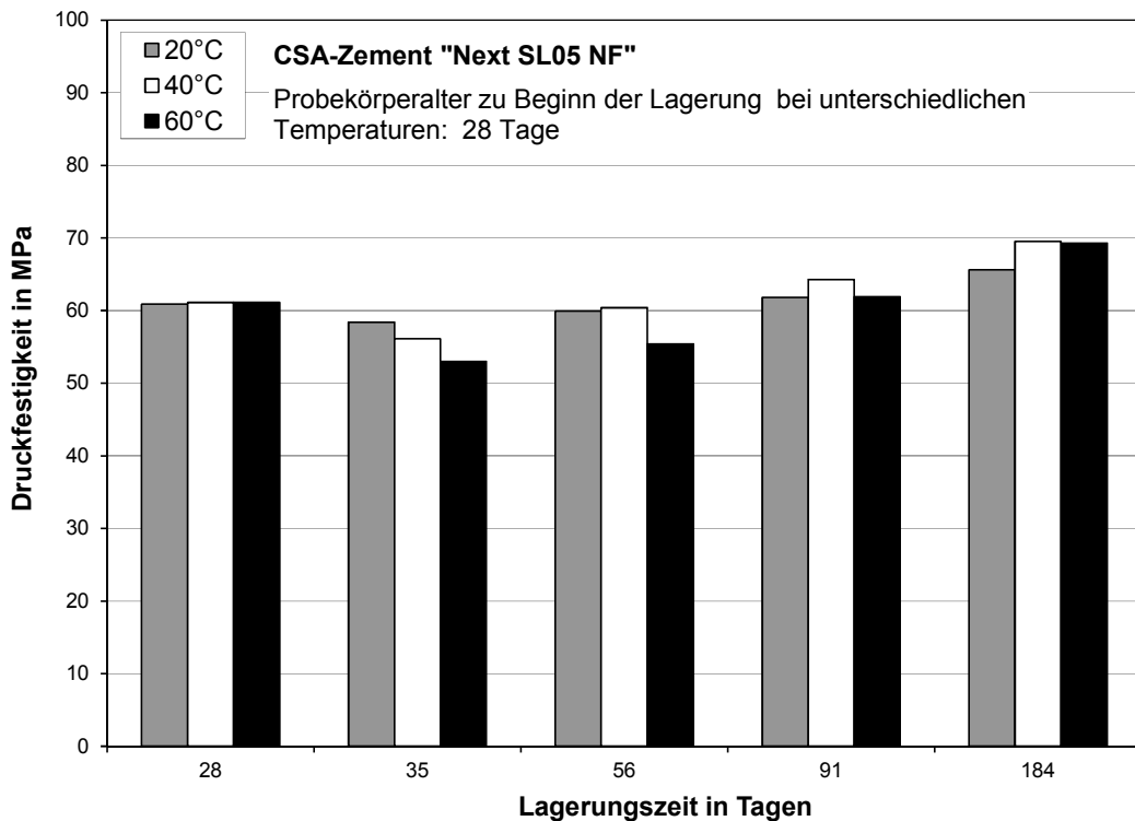
Bild 1: Mörteldruckfestigkeit mit schnellerhärtendem Zement auf Basis von Calciumaluminatsulfat "Next SL05 NF" bei 20 °C, 40 °C und 60 °C
