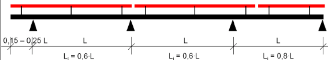
Bild 11: Ideale Stützweite
