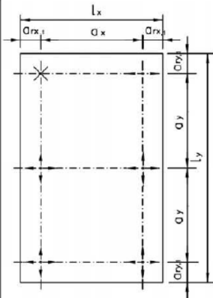
Bild 13: Fassadenplatte mit 6 Agraffen – Lagerungsart 2
