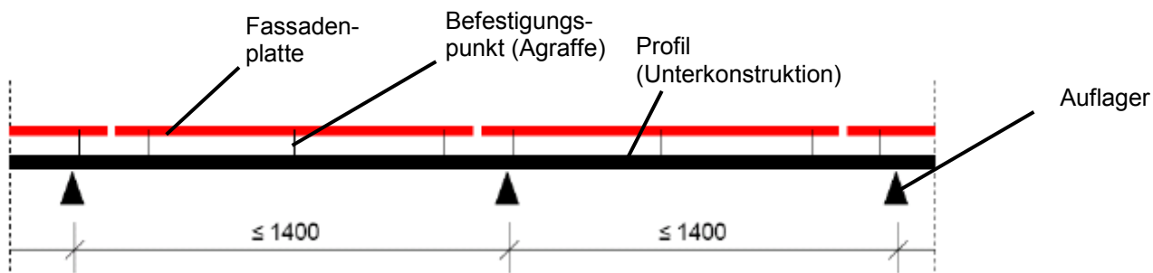
Bild 9: Die Auflager von Schienen, auf denen sich 3 Befestigungspunkte einer Platte befinden, haben einen maximalen Abstand von 1.4 m.
