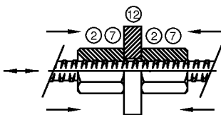
Bild 9 Ø12 - 32
