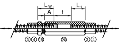
Bild 10 Muffenstoß - Spannschloß Ø12 - 32
