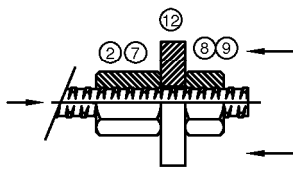
Bild 5 Ø12 - 32
