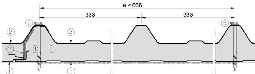
Obergurtbefestigung
