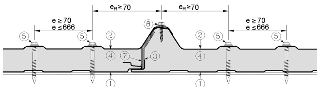
Untergurtbefestigung
