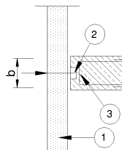
BILD 3 Beton-Auflager
