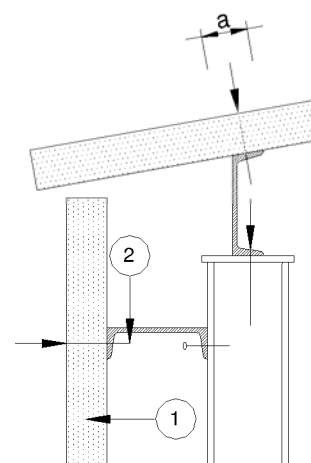
BILD 6 Traufpunkt Wandpaneel
