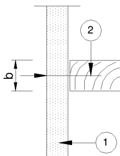
BILD 2 Holz-Auflager
