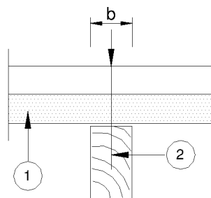
BILD 2 Holz-Auflager
