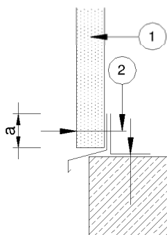
BILD 4 Fußpunkt Wandpaneel aufgesetzt
