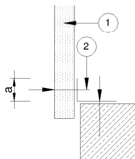
BILD 5 Fußpunkt Wandpaneel vorgesetzt
