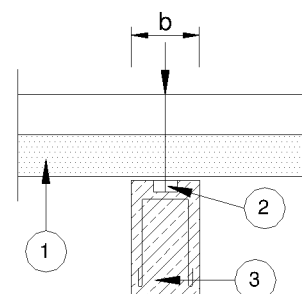
BILD 3 Beton-Auflager
