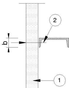
BILD 1 Stahl-Auflager
