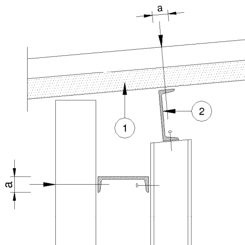
BILD 4 Traufpunkt
