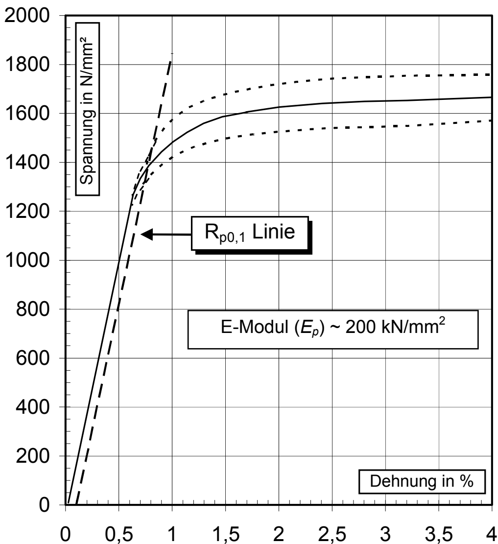
Bild 2: Spannungs - Dehnungslinie
