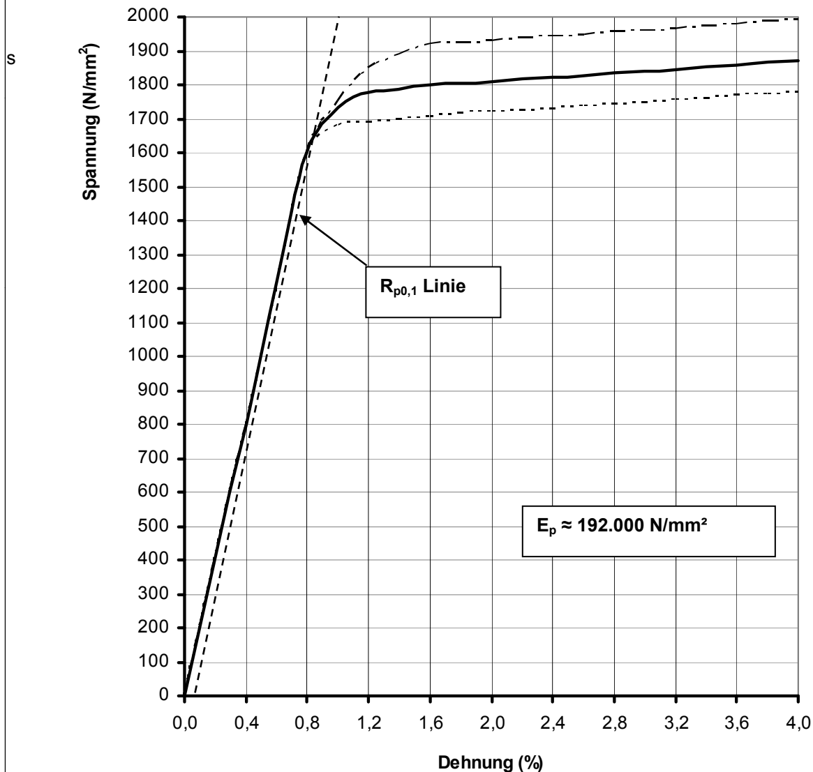
Bild 2: Spannungs - Dehnungslinie
