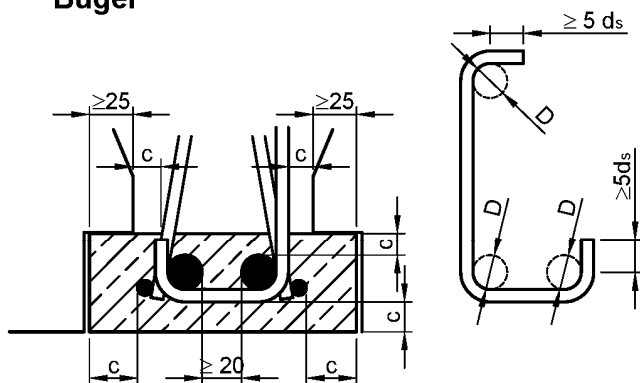
Bild 17: D- / E-Träger mit Betonfußleiste und einschnittigen Bügel
