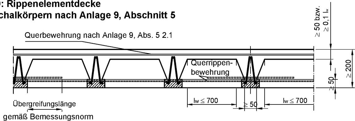
Bild 10: Rippelementdecke mit Betonschalung nach Anlage 9, Abschnitt 5
