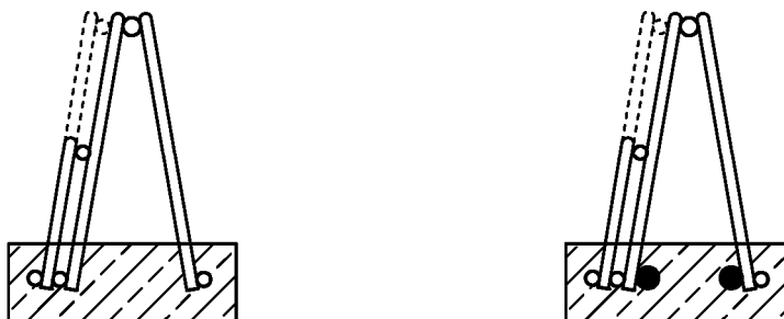
Bild 23: DH- bzw. EH-Gitterträger als Verbund- und Schubzulagen
