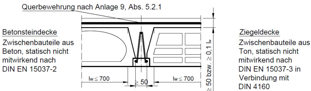
Bild 8: Rippendecke nach Anlage 9, Abschnitt 5
