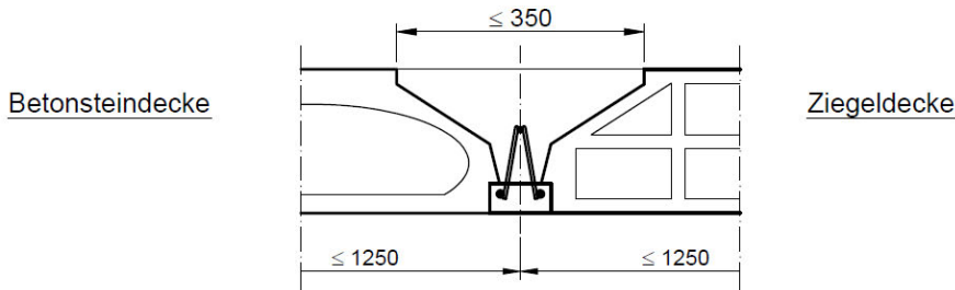
Bild 6: Rippendecke nach Anlage 9, Abschnitt 5
