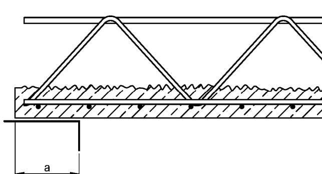
Bild 19: Auflagerung ohne Montageunterstützung am Rand
