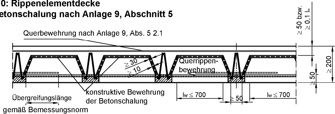
Bild 11: Elementrippendecke nach Anlage 9, Abschnitt 5
