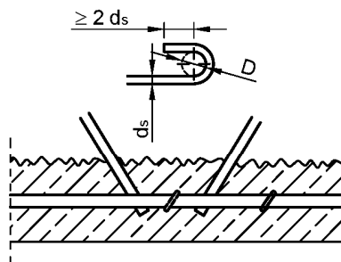
Bild 14: Querbügel
