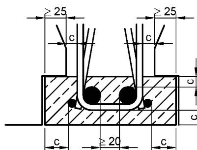
Bild 18: D- / E-Träger mit Betonfußleiste und zweischnittigen Bügel
