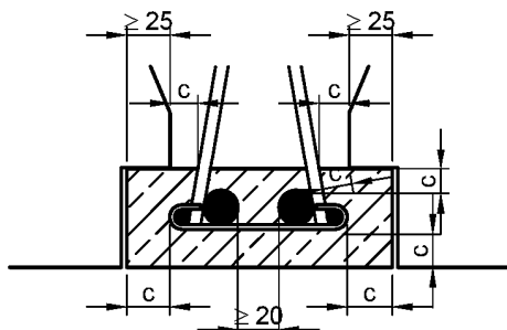
Bild 15: D- / E-Träger mit Betonfußleiste und Querbügelleitern
