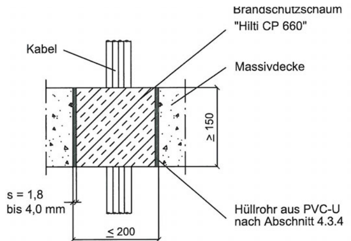
Schnitt Y-Y
