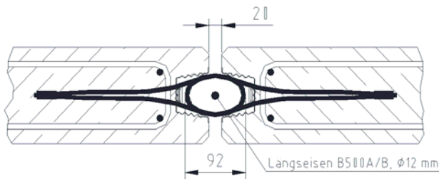
Bild 11: Regeldetail Fuge
