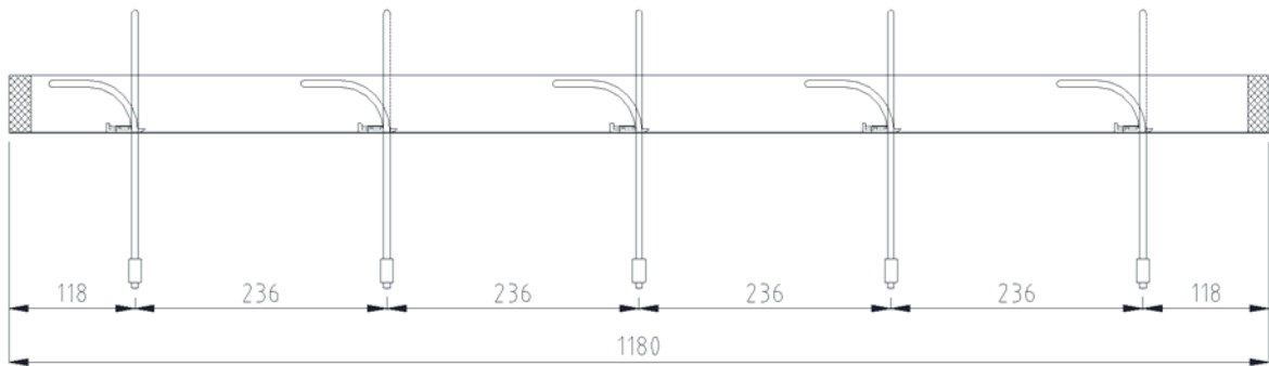
Bild 1: VS ® -BZ-50 (Längsschnitt)
