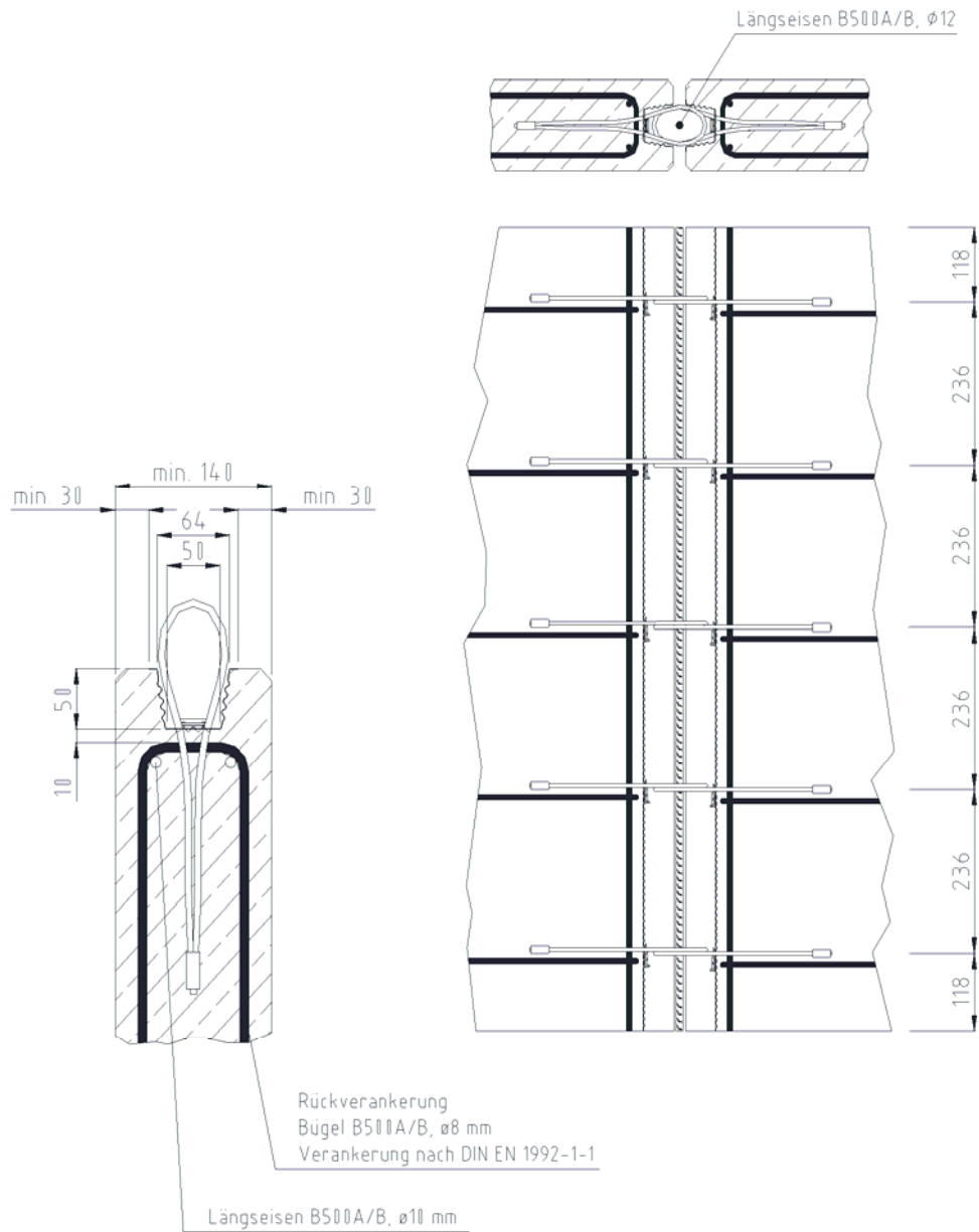
Bild 10: Vergussnut, Bewehrung
