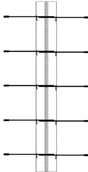
Bild 14: Regelfall Schlaufenüberlappung
