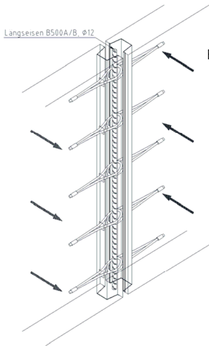
Bild 19: Kombinierte Beanspruchung
