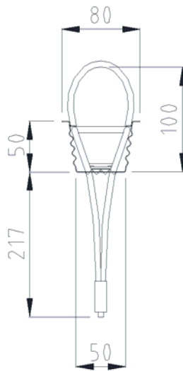
Bild 2: VS ® -BZ-50 (Querschnitt)
