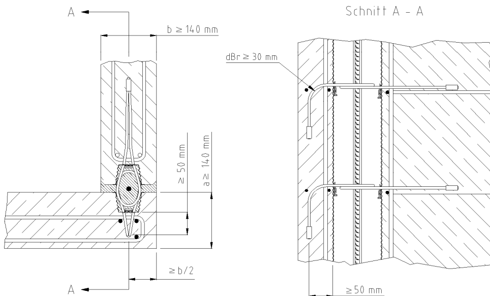
Bild 7: Wand – Wand – Eckverbindung - Detail bei abgewinkelter Seilschleufe
