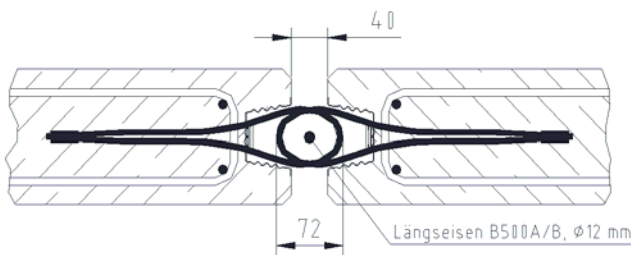
Bild 13: Maximale Fugenbreite
