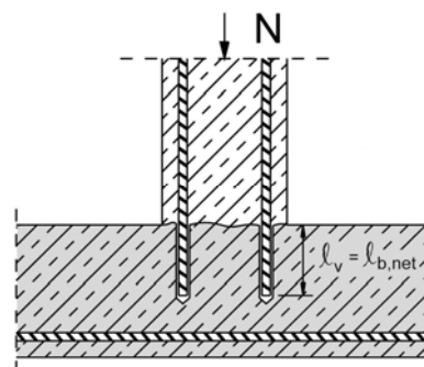
Bild 4: Bewehrungsanschlüsse überwiegend auf Druck beanspruchter Bauteile
