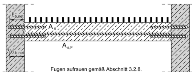
Bild 3: Endverankerung von Platten oder Balken, bemessen als Einfeldträger
