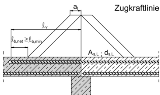
Bild 5: Verankerung von Bewehrung zur Deckung der Zugkraftlinien.
