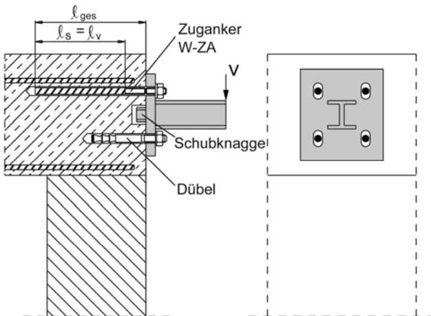
Bild 8: Übergreifungsstoß für die Verankerung von ausragenden Bauteilen
