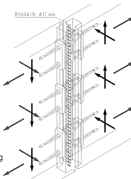
Bild 17: Beanspruchung senkrecht zu Fugenlängsrichtung und Wandebene
