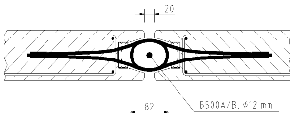
Bild 10: Regelfall Fuge
