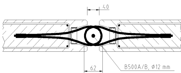
Bild 12: Maximale Fuge
