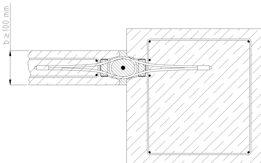
Bild 4: Stützen - Wandverbindung
