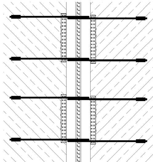
Bild 13: Regelfall Schlaufenüberlappung
