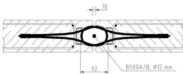
Bild 11: Minimale Fuge
