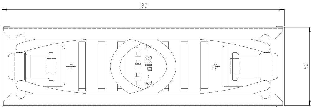
Bild 2: Draufsicht auf die geöffnete Box und die eingeklappten Seilschlaufen
