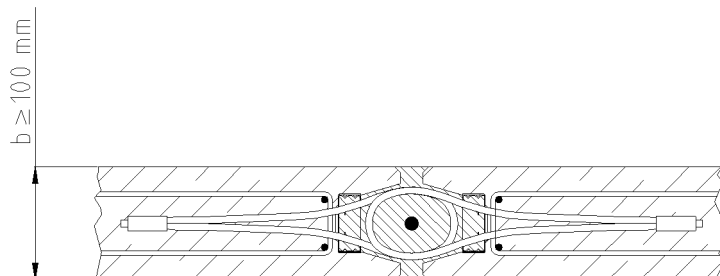
Bild 3: Wand - Wandverbindung
