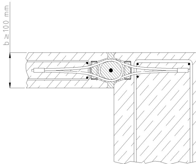
Bild 5: Wand – Wand – Eckverbindung - Regeldetail
