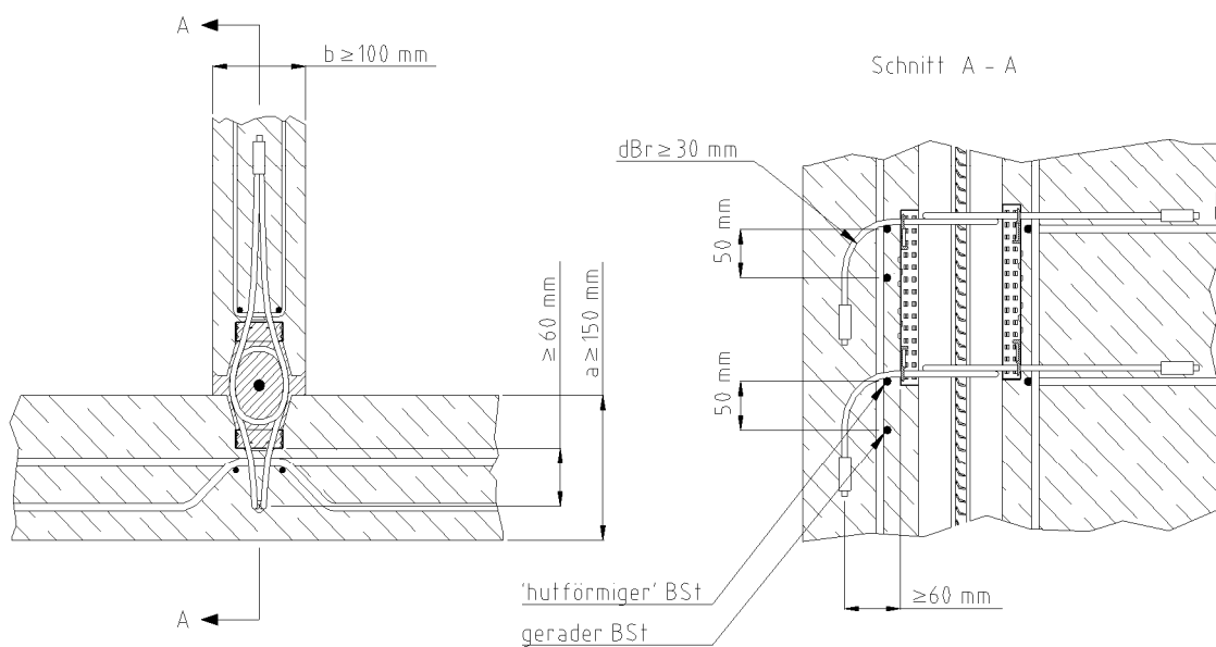
Bild 8: Wand – Wand – T-Verbindung - Detail mit abgewinkelten Seilschlaufen
