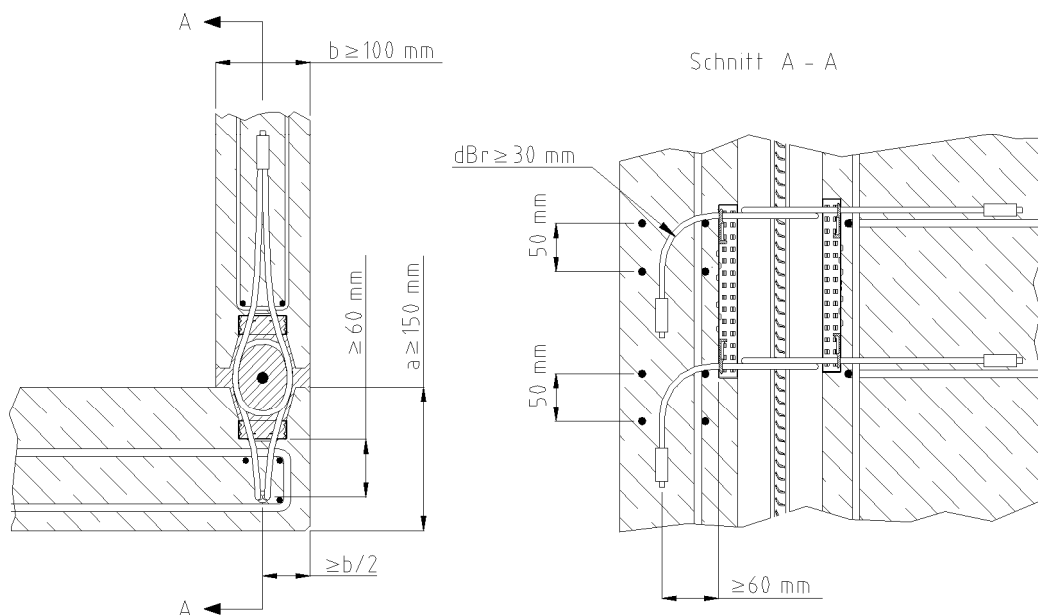
Bild 6: Wand – Wand – Eckverbindung - Detail mit abgewinkelten Seilschlaufen
