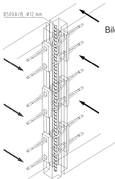
Bild 18: Kombinierte Beanspruchung
