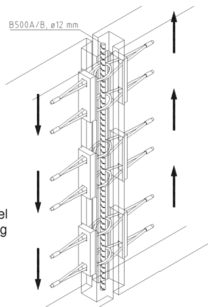
Bild 17: Beanspruchung senkrecht zu Fugenlängsrichtung und Wandebene
