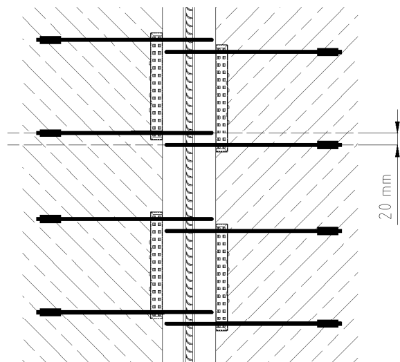
Bild 14: Maximale vertikale Fehllage: 20 mm
