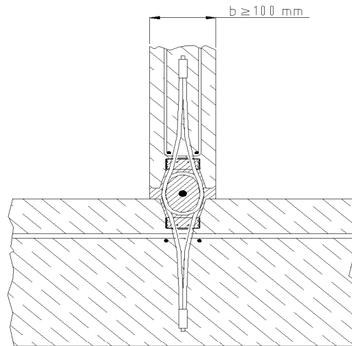
Bild 7: Wand – Wand – T-Verbindung - Regeldetail
