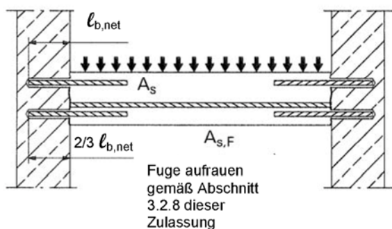
Bild 5: Verankerung von Bewehrung zur Deckung der Zugkraftlinien
