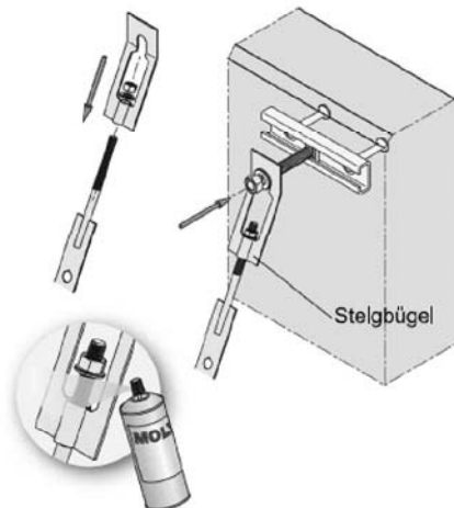
D1' Montieren des Stelgbügels an der Gewindestange des Lochbandes mit Muttern und U-Scheiben. Bei Typen FPA -5Z, -5A und -5AZ wird empfohlen, den Stelgbügel bzw. die obere Befestigung vor der Montage als Schablone für die richtige Platzierung der Bohrlöcher (Dübelbefestigung) zu verwenden. Fassadenplatte mit vor- montiertem FPA-5-Montageteil an gesetztem Dübel oder Halfen- schlene befestigen. Molykote® HSC-Spray auftragen und Fertigteil am Stelgbügel justieren. Während des Justierens hängt das Fertigteil noch am Kranhaken.
