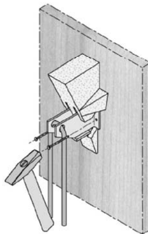
C3 Rohbauteil mit Nägeln an Schalung befestigen.
